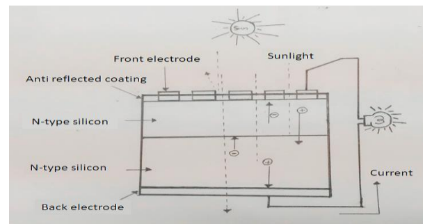
Fig. PV cell
